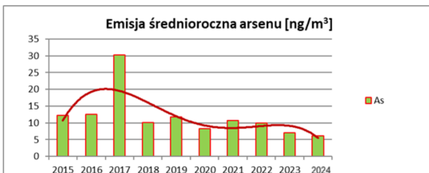
WYKRES 15: Emisja średnioroczna arsenu.
