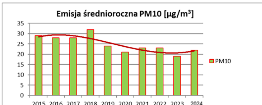
WYKRES 12: Emisja średnioroczna PM10
