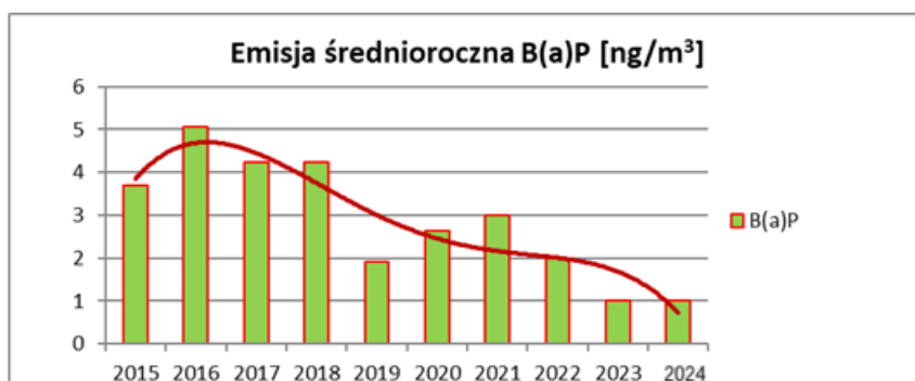
WYKRES 14: Emisja średnioroczna B(a)P.
